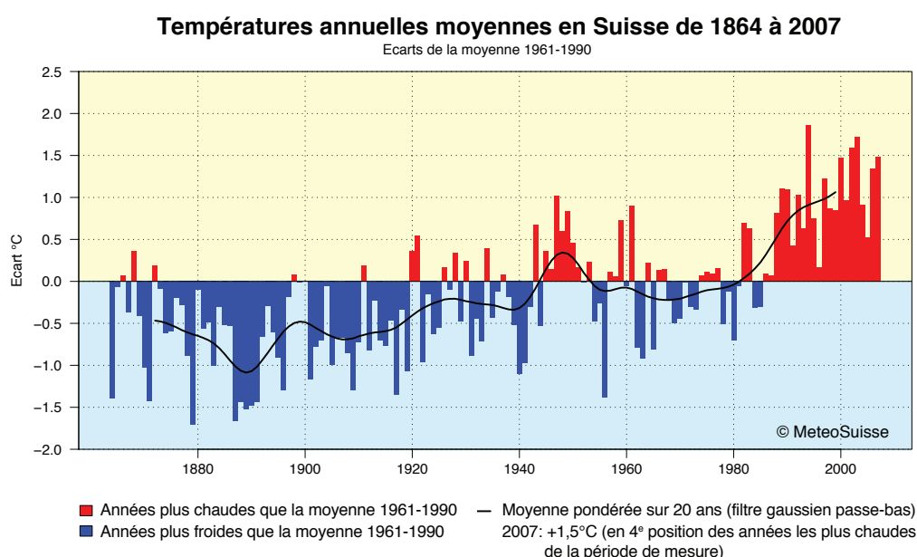
Figure 1: Ecart des températures annuelles moyennes en Suisse par rapport à la période de comparaison 1961 -1990 (écarts positifs en rouge, négatifs en bleu). Le graphique présente les moyennes de douze stations de mesure situées à différentes altitudes en Suisse septentrionale et méridionale (source: MétéoSuisse, 2008).
