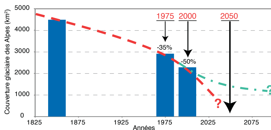
Figure 3: Le glacier de Tschirva et ses moraines du 19 e siècle («petit âge glaciaire») et l'avenir des glaciers des Alpes: l'évolution de la surface totale estimée des glaciers alpins indique que le processus de fonte s'est déjà fortement accéléré et que son déroulement au cours des premières décennies du 21 e siècle pourrait être dans une large mesure et pour longtemps irréversible. Données et extrapolations d'après Zemp et al. (2006) et Haeberli et al. (2007).
