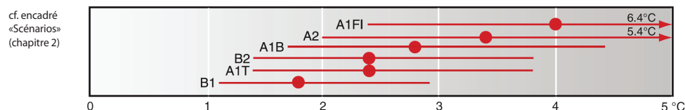
Figure 1: Relations entre le réchauffement moyen de la Terre par rapport à aujourd'hui comme indicateur de changements climatiques et ses principaux impacts sur différents secteurs. A noter qu'aucun des scénarios RSSE d'émission du GIEC mentionnés dans le graphique du bas n'a été privilégié, mais que seuls sont indiquées les relations entre les changements de la température globale moyenne et leurs impacts sans adaptation (tiré de GIEC, 2007c, figure 3.6, p. 51).
